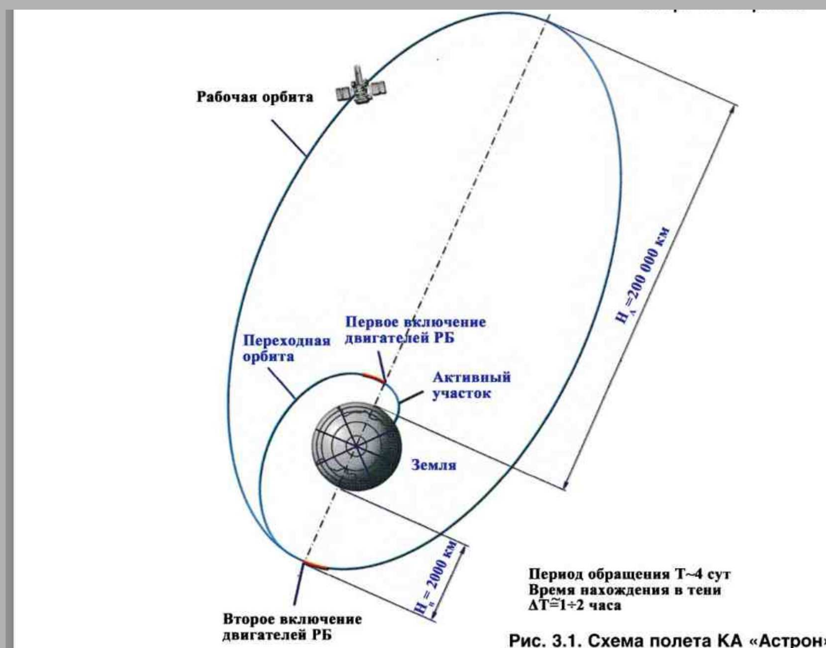
Рис. 3.1. Схема полета КА «Астрон»
